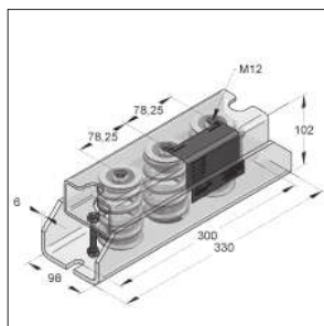
FL rugós tartó 2 típusú ház
