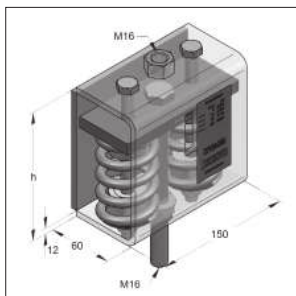
FH2 rugós tartó
