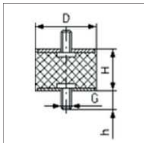
KK típusú hengeres gumirugó
