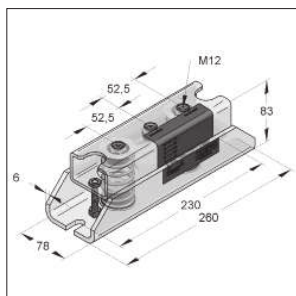
FL rugós tartó 1 típusú ház
