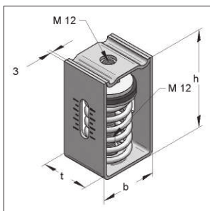
FH1 rugós tartó
